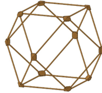
Kuboktaeder
