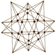
Dodekaederstern
