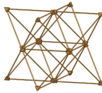
Oktaederstern
